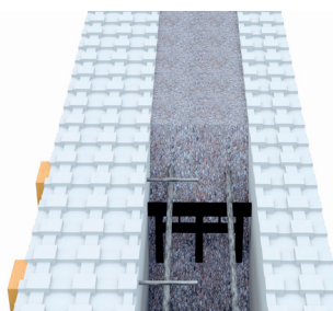
FinnEPS-harkkoseinään kiinnittäminen
